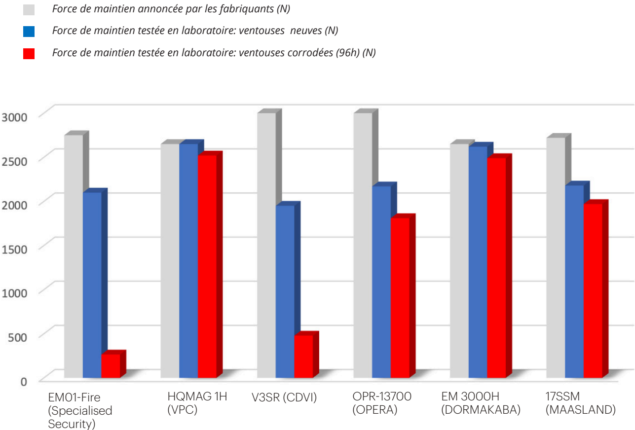
Figure 1: Graphique de la force de maintien annoncée, testée et corrodée des ventouses électromangétiques apparentes
